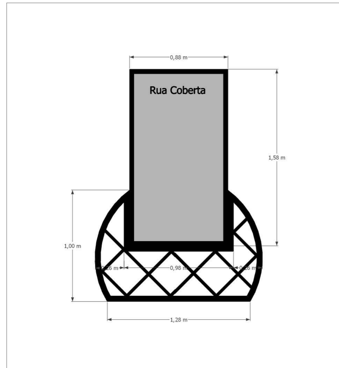
- VISTA FRONTAL
