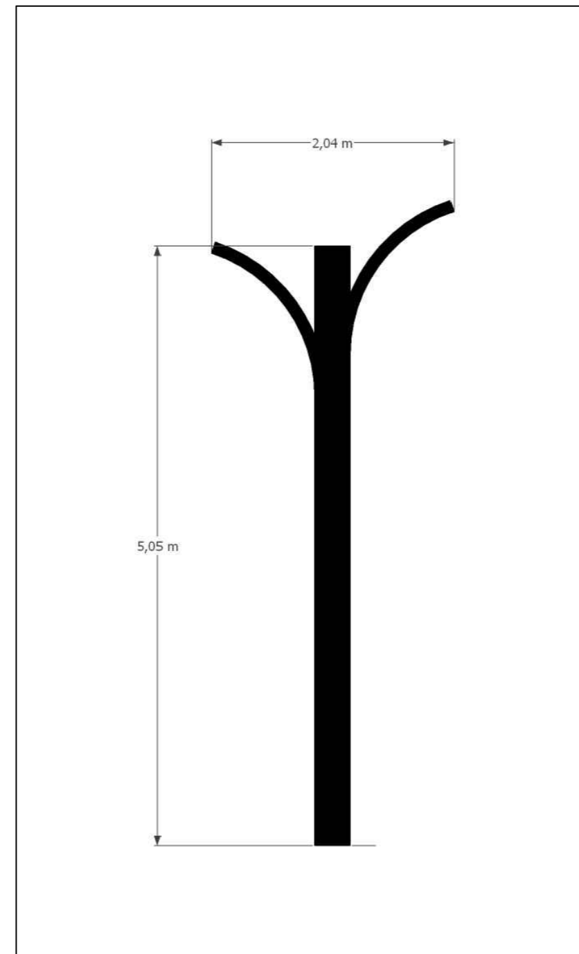
- PILAR TIPO 2, VISTA FRONTAL
