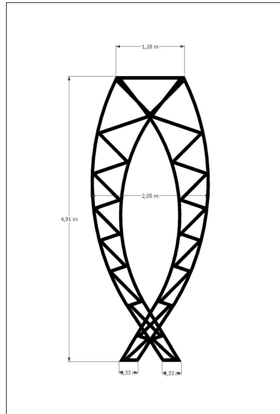
- PILAR TIPO 1, VISTA FRONTAL
