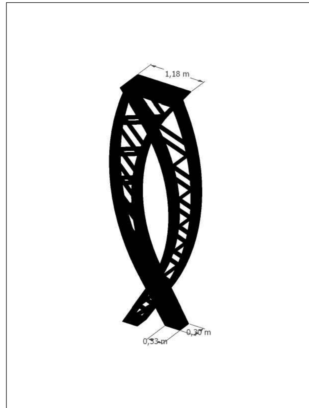
- PILAR TIPO 1, PERSPECTIVA
